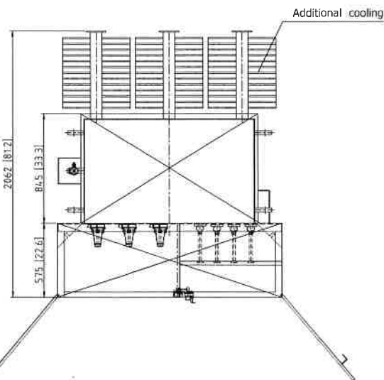
L.V. TERMINAL
