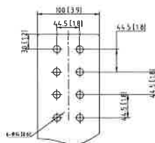
L.V. TERMINAL
